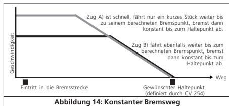
Abbildung 14: Konstanter Bremsweg
