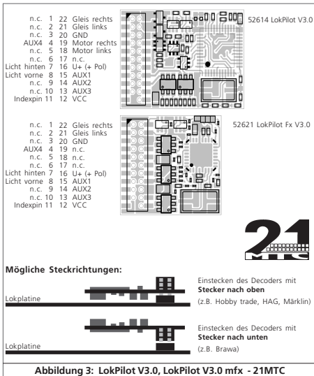
Abbildung 3: LokPilot V3.0, LokPilot V3.0 mfx - 21MTM
