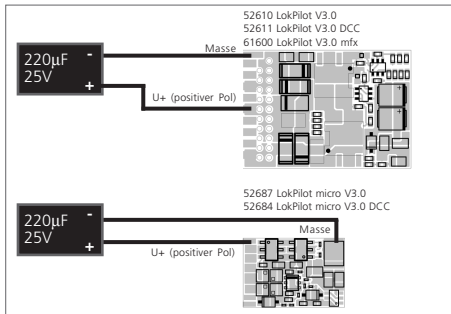
Abbildung 10: 220 µF Kondensator an LokPilot, LokPilot micro
