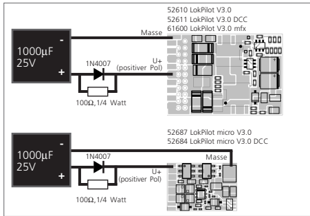
Abbildung 11: 1000µF Kondensator an LokPilot, LokPilot micro
