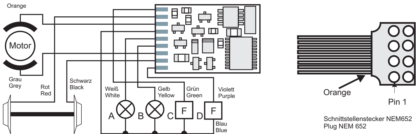
Anschluß des LE1025A / Wiring the LE1025A
