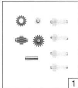
Getriebe Nachrüstsatz Gear expanding set Jeu d'engrenage complémentaire
